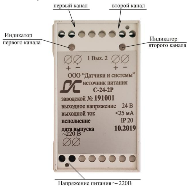
Рис. 1 – расположение разъемов ИП.
