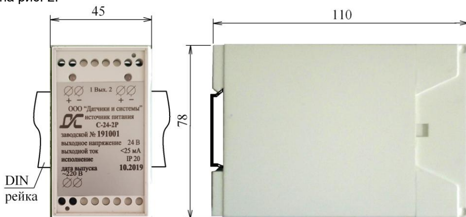
Рис. 2 – положение ИП при монтаже и его габаритные размеры.
