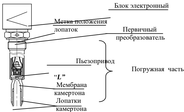
Рисунок 2 – Схема СУ
