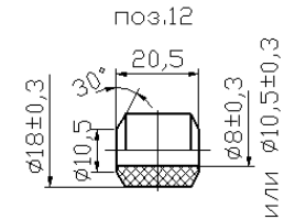
Кольца уплотнительные (варианты)
