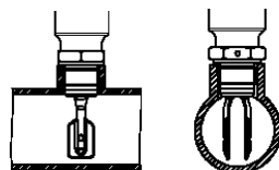
Рисунок 8 -Положение лопаток СУ в трубе
