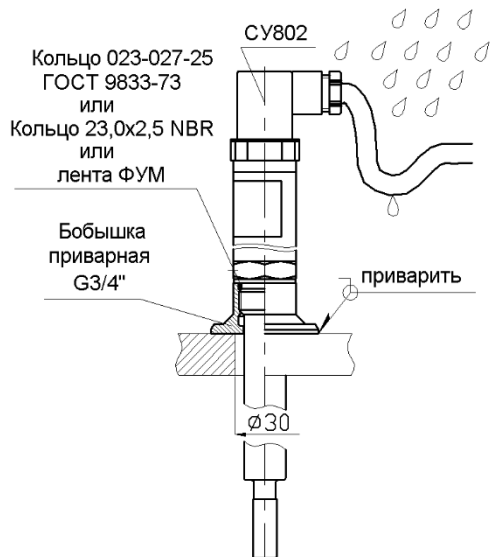
Рисунок А.2 – установка СУ
