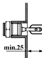
Рисунок 9 -Положение камертона в емкости
